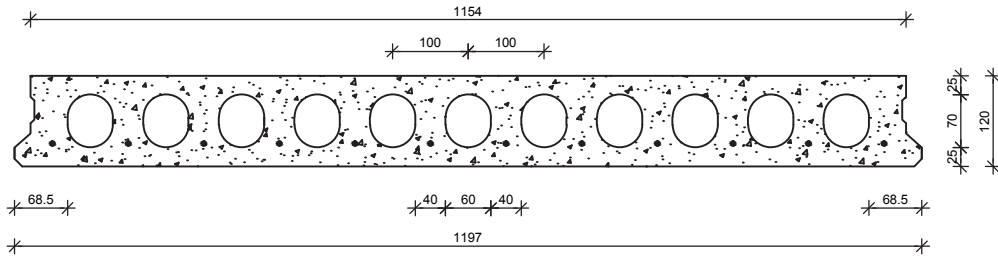
TOPFLOOR 120mm DEEP SLAB
